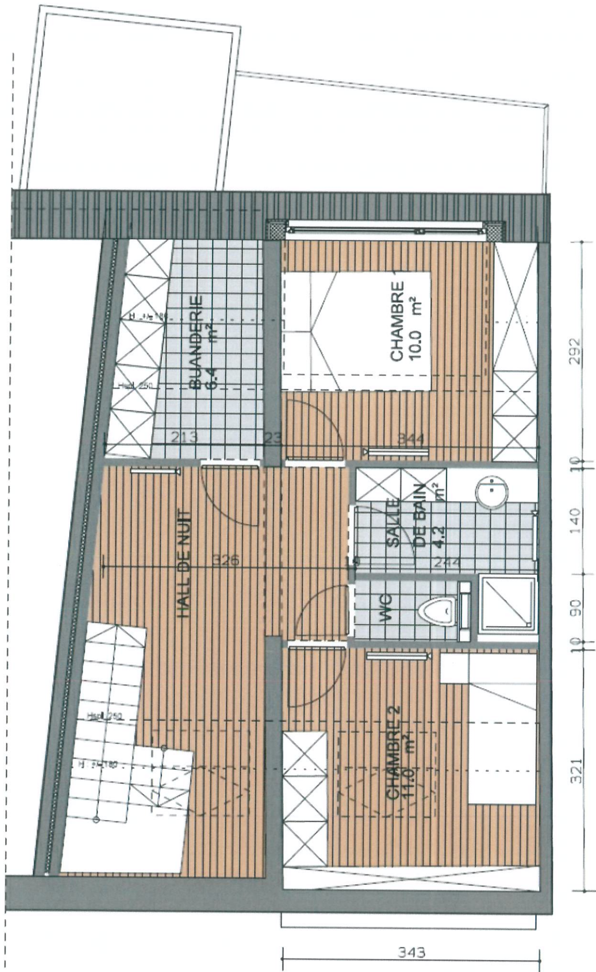
PLAN NIVEAU +2
