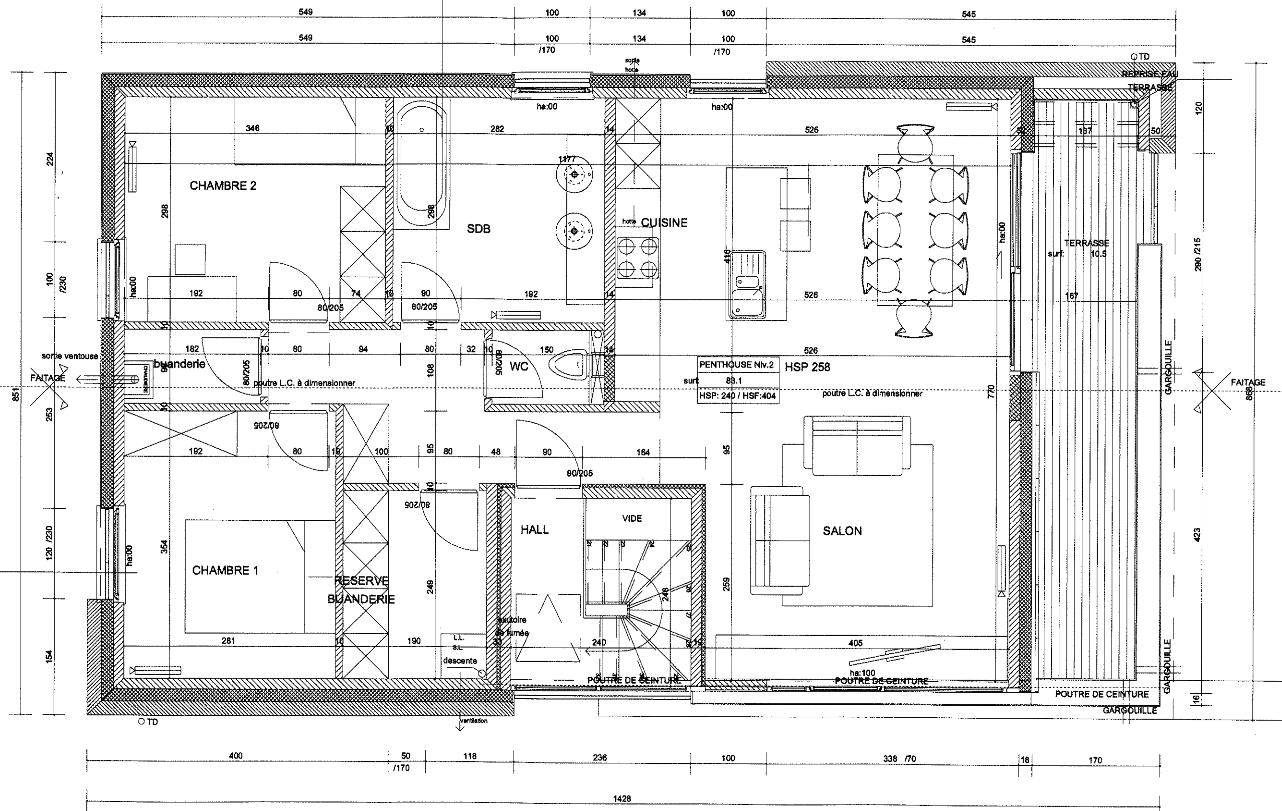
PLAN ETAGE 2ème
